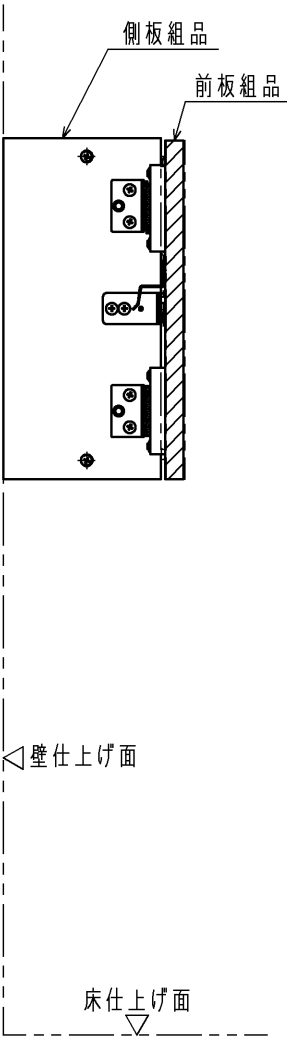
A - A キャビネット側
